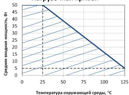
Нагрузочная кривая
