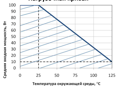
Нагрузочная кривая
