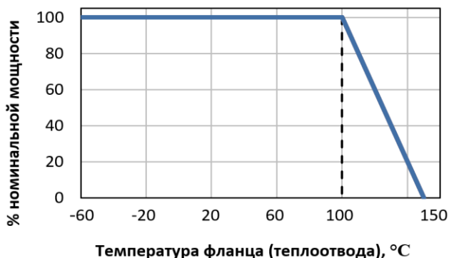
Нагрузочная кривая
