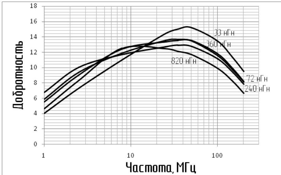
КИФ1608
