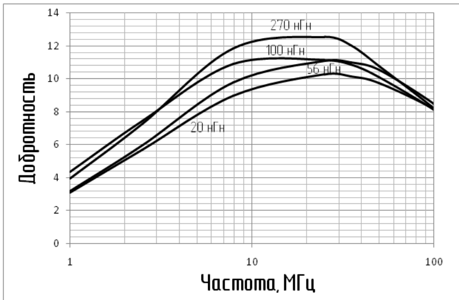
КИФ1005
